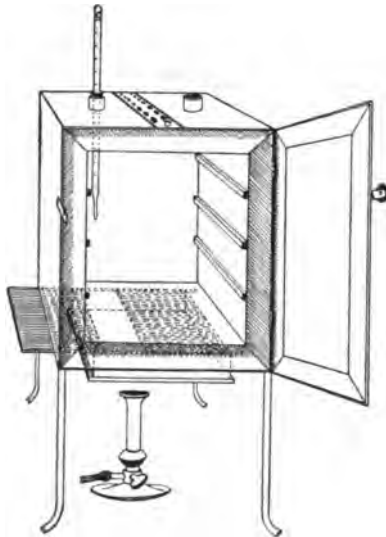
FIG. 26.—Hot-air oven.
